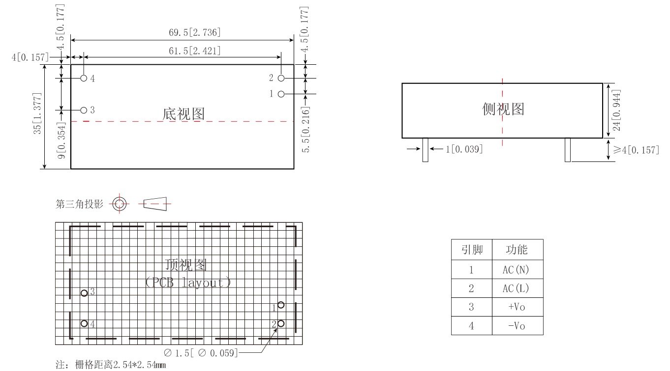
标准式封装
