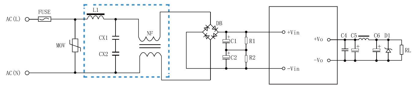
外部电路元器件的典型值
