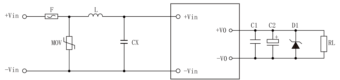
外部电路元器件的典型值
