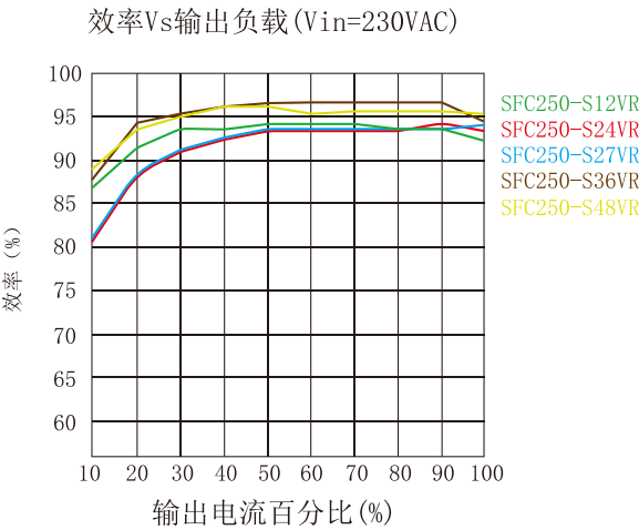
效率曲线图
