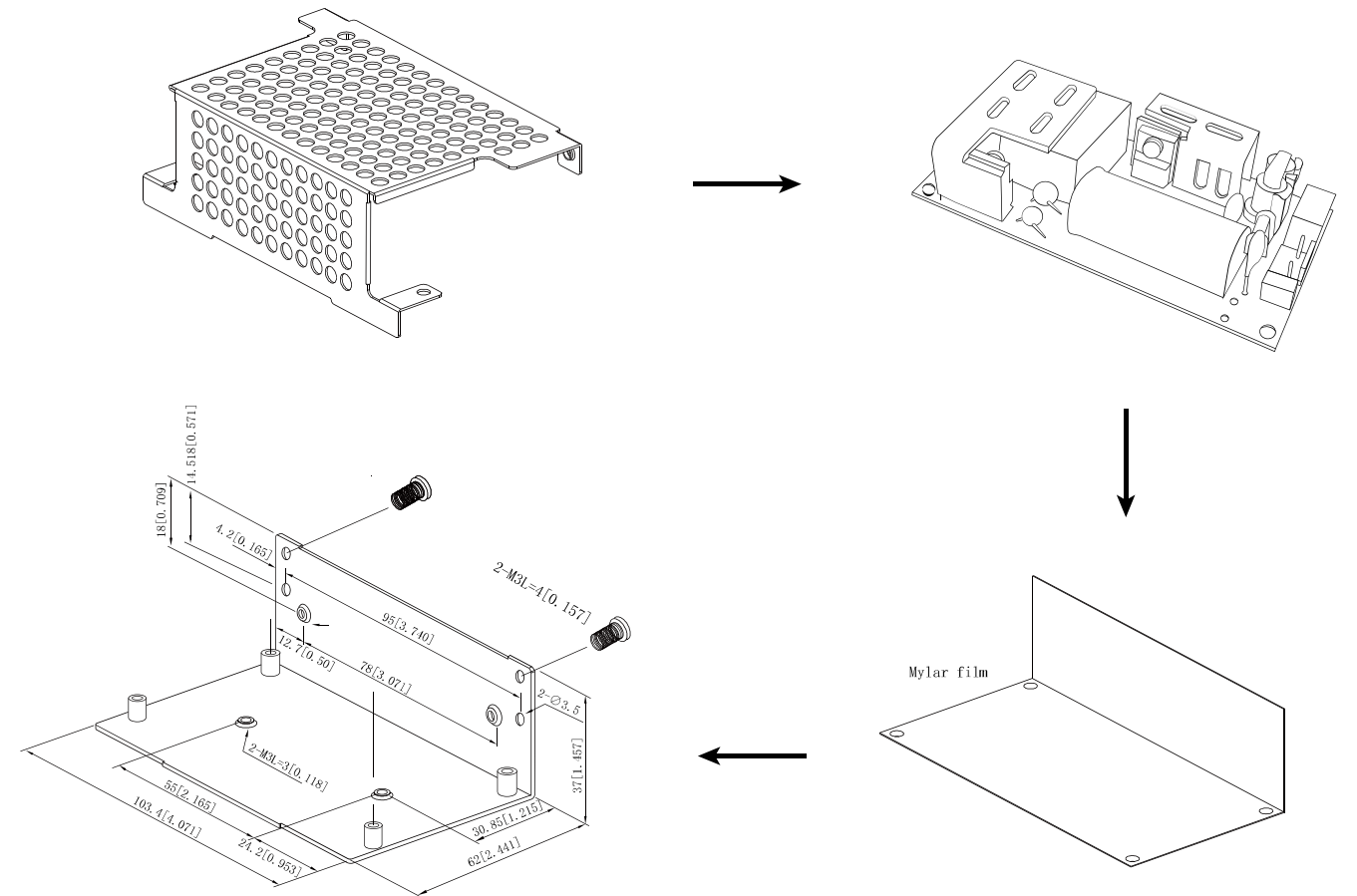
机壳型 (C) 封装尺寸
