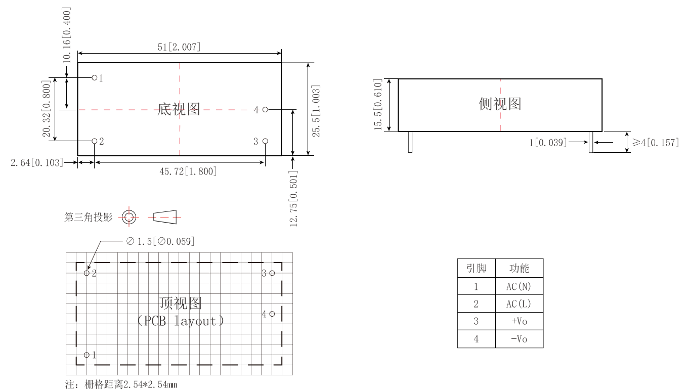
标准式封装
