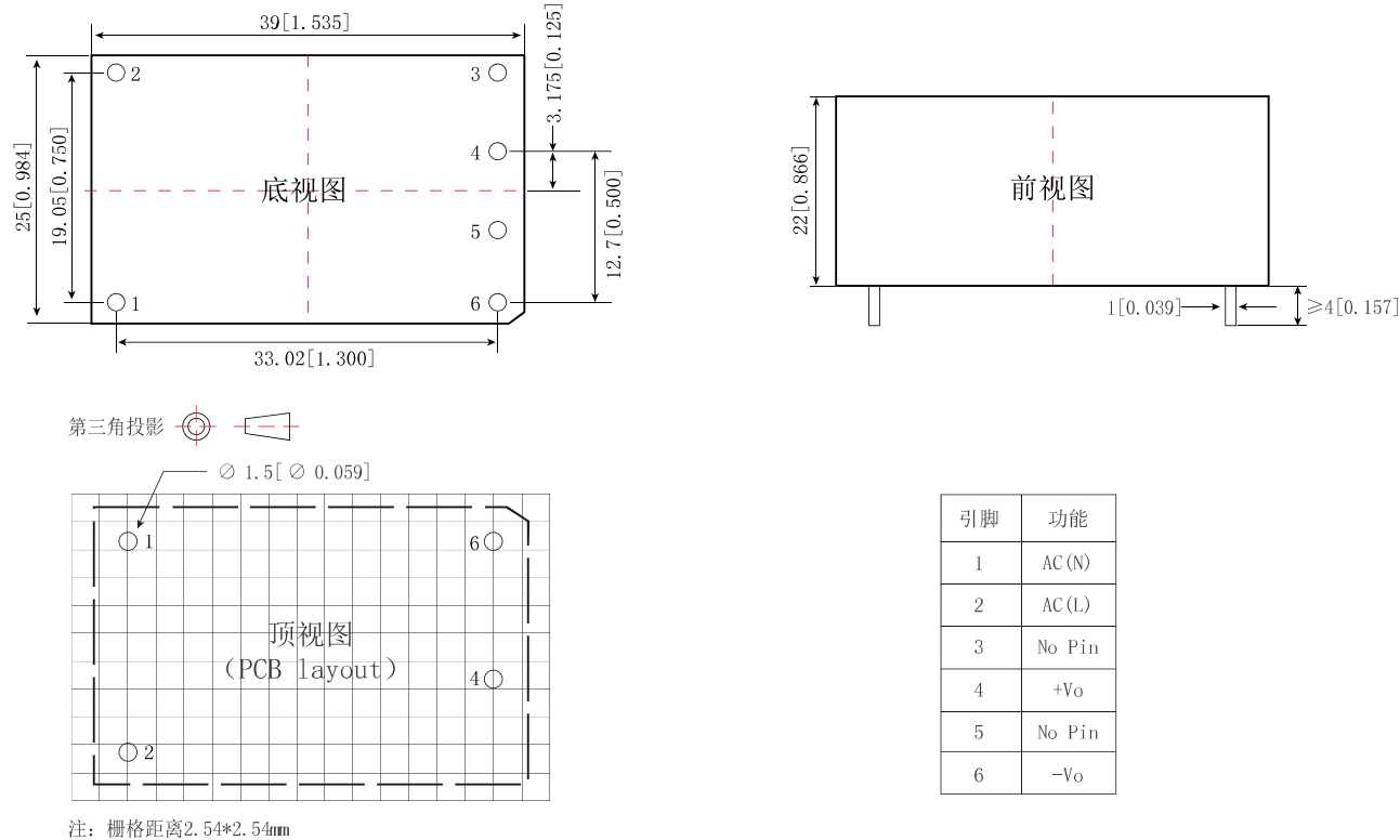
标准式封装
